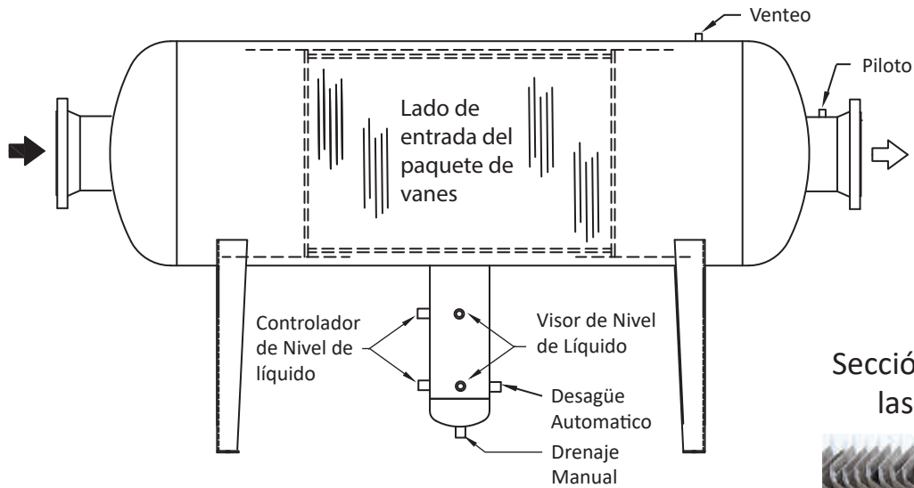
Tipo 100H con bota para la retención de líquidos
