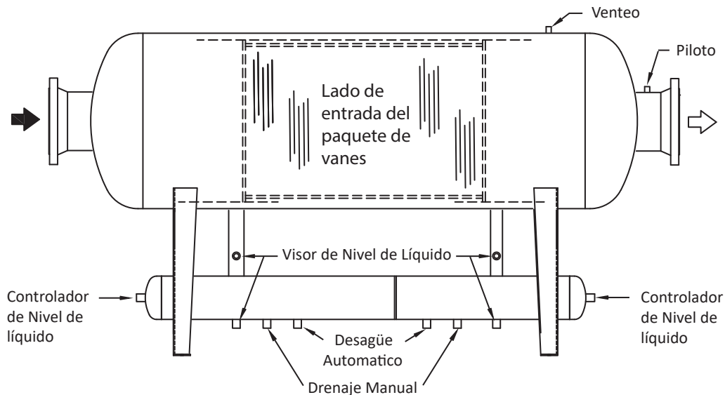
Tipo 100H con barril horizontal para la retención de líquidos
